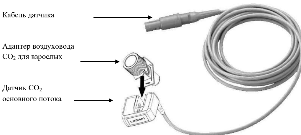
Рисунок 13.3.1 – Демонстрация подключения датчика CO 2 основного потока
