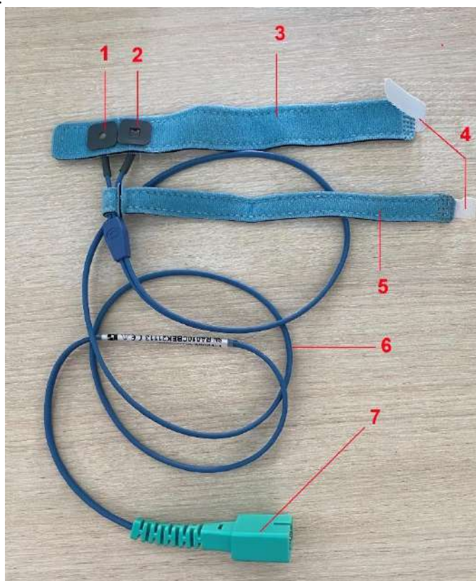
Рисунок 2.2.18 – Датчик пульсоксиметрии для новорожденных
