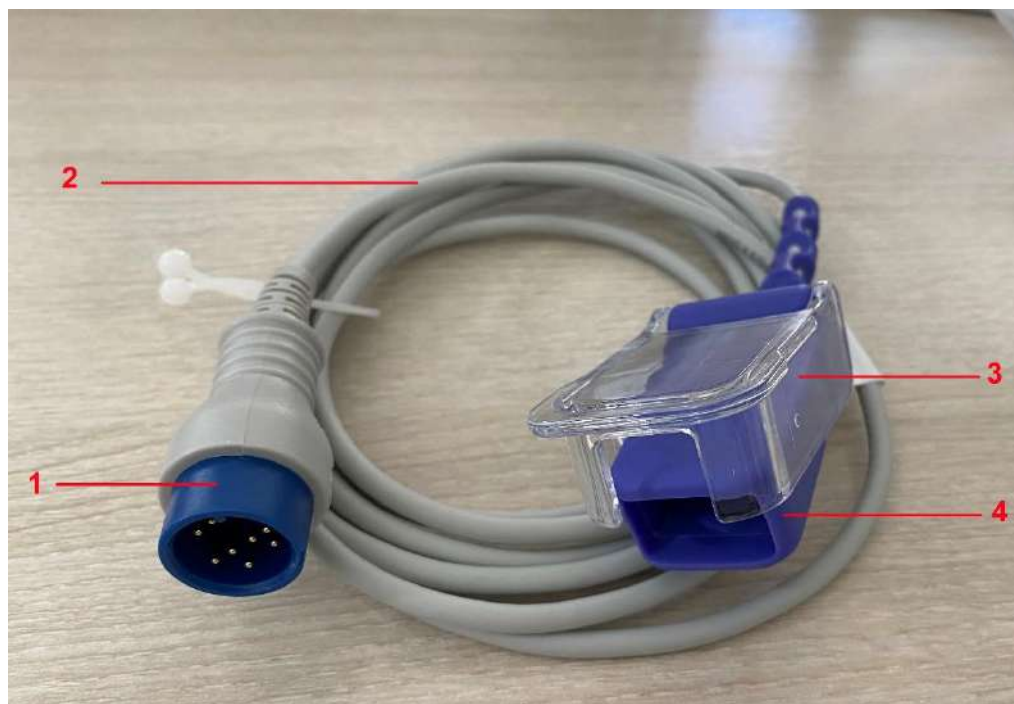
Рисунок 2.2.1 – Кабель внешний
