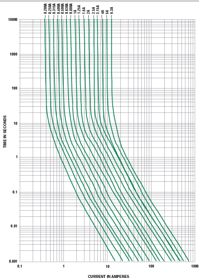
Рисунок 4.1.1 – Кривая времени срабатывания предохранителя в секундах (по вертикали) в зависимости от величины тока в амперах (по горизонтали).
