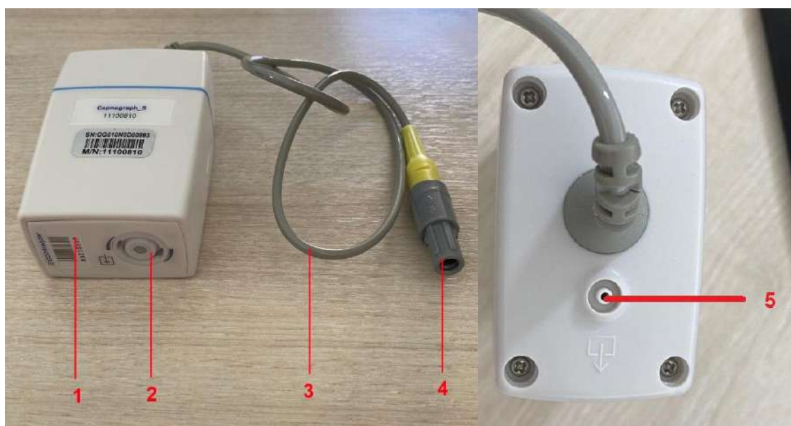
Рисунок 2.2.11 – Датчик CO 2 бокового потока
