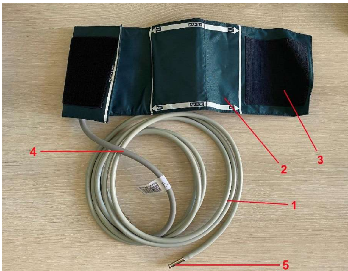
Рисунок 2.2.3 – Манжета НИАД (Манжета НИАД для детей отличается только размером манжеты, конструкция – аналогична)
